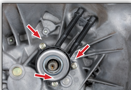
Fig. 7: Montaje del nuevo dispositivo central de desembrague
